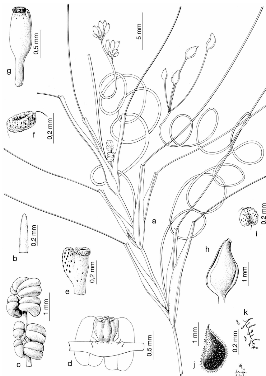
Lám. 22.— Ruppia drepanensis , Doñana, Las Marismillas, Huelva (SEV 38201): a) tallo con hojas, inflorescencias y frutos; b) ápice de una hoja; c) inflorescencia, sin pedúnculo; d) flor joven, antes de desprenderse uno de los estambres; e) carpelo; f) estigma; g) carpelo fecundado, antes de la fructificación; h) drupa; i) zona estigmática, en la fructificación; j) drupa antes de la germinación, con restos del pericarpo; k) detalle de la superficie de una drupa antes de la germinación.
